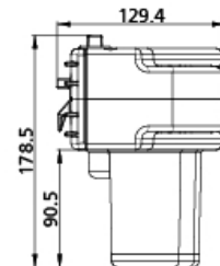
Seitenansicht Side view
