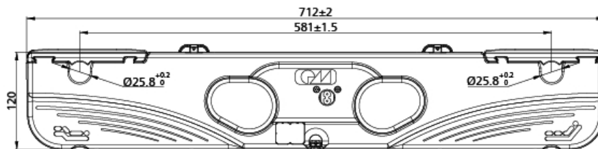
Draufsicht Top view
