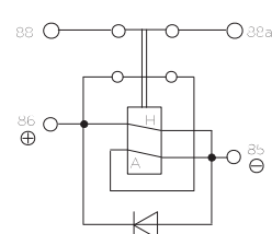
Suppression diode
